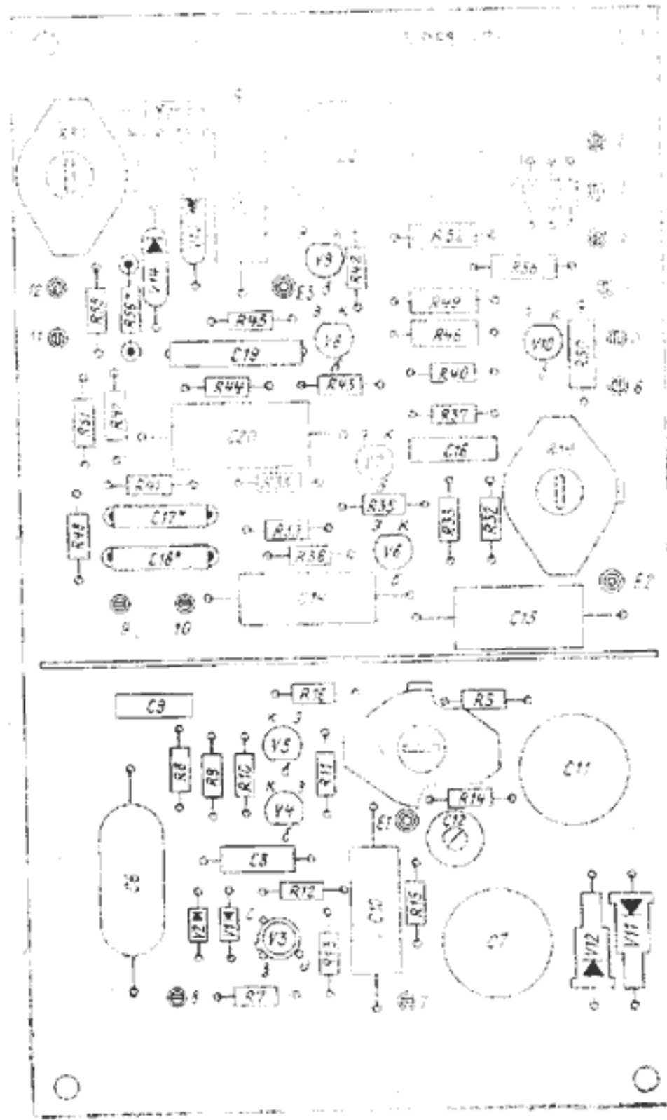
Блок комбинированный
